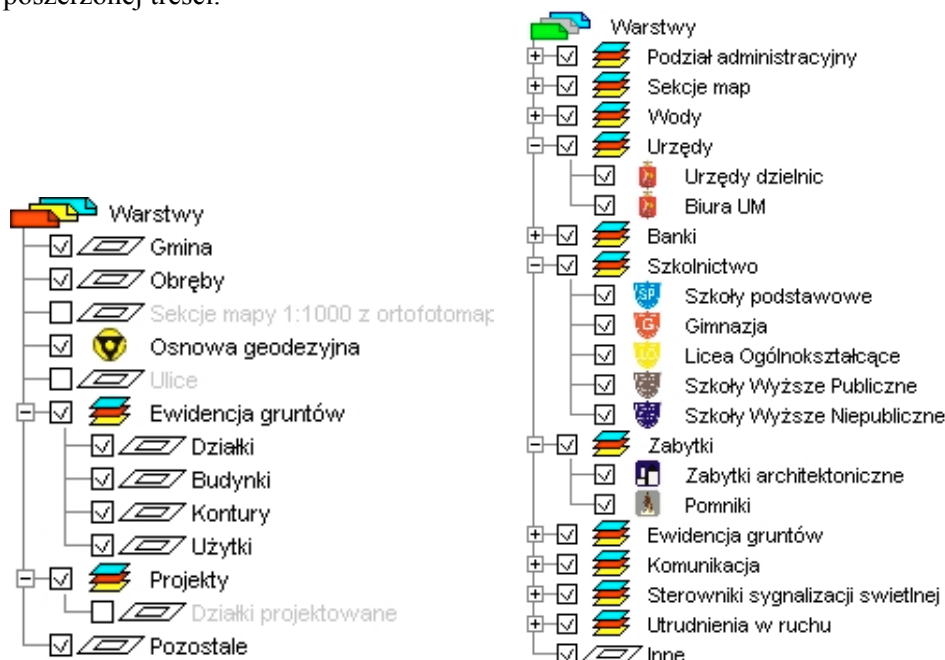
Rys. 4. Przykład typowego i rozszerzonego zestawu warstw informacyjnych
