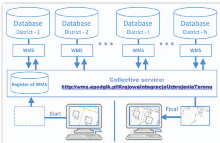
Rys. 1. Koncepcja zbiorczej usługi WMS do prezentacji uzbrojenia terenu
